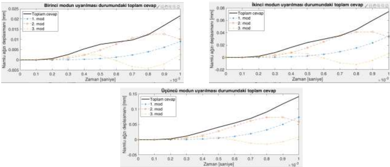
Şekil 6. Titreşim modlarının namlu ağız deplasmanına etkisi
