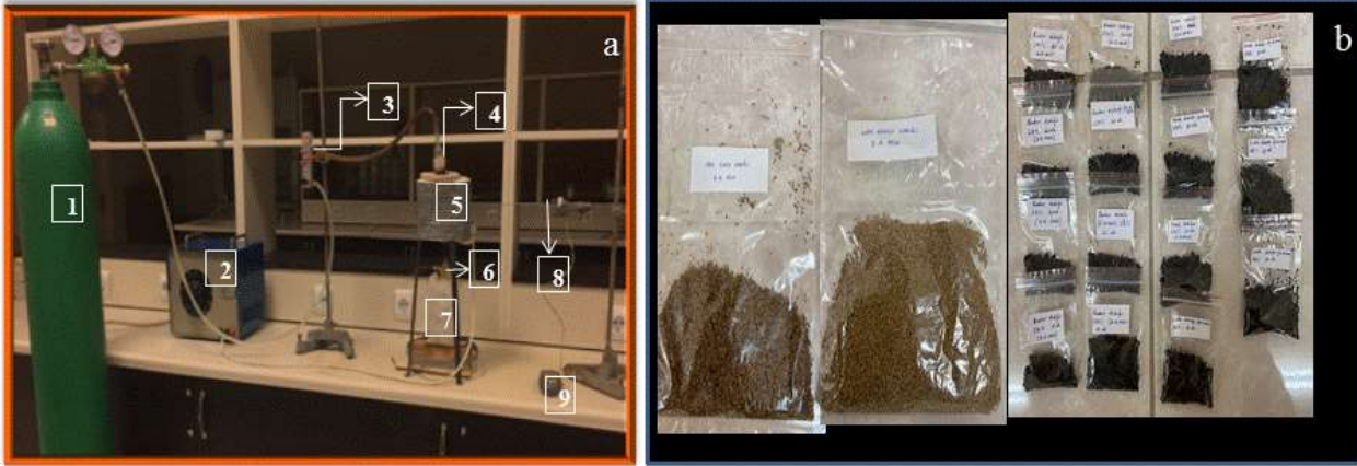
Şekil 1. a) Torrefaksiyon deney sistemi: 1. Azot tüpü, 2. Değişik voltaj transformatörü, 3. Rotametre, 4. Cam reaktör, 5. Silindirik fırın, 6. Sıvı ürün toplama kabı, 7. Buz banyosu, 8. Termocift, 9. Termocift okuyucu
