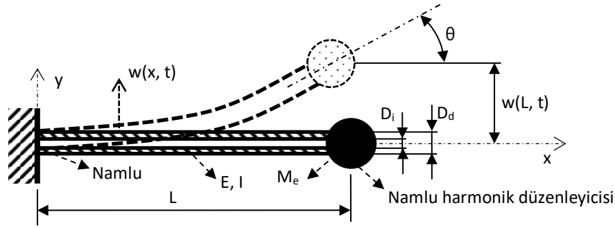
Şekil 5. Ankastré çubuk olarak modellenen namlu ve namlu harmonik düzenleyicisi
