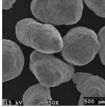
Şekil 7. Bilyalı dövme işleminde kullanılan bilyaların SEM görüntüsü
