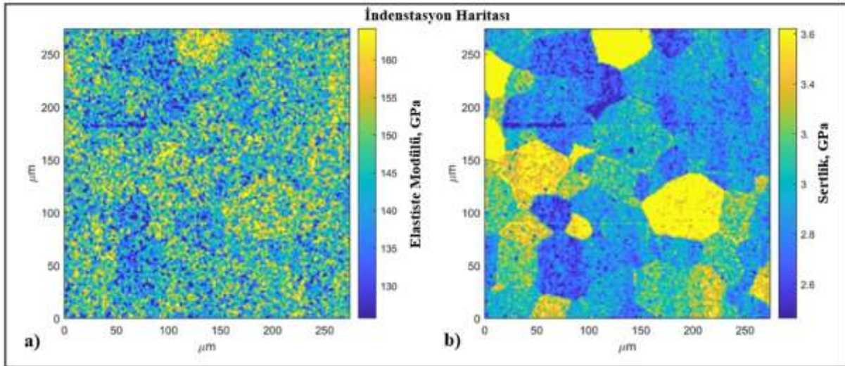
Şekil 4. Ticari saflıktaki titanyum alaşımının a) elastisite modülü, b) sertlik haritası (Magazzeni et al., 2021)
